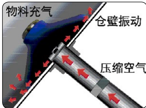
料斗剖面，显示流化器使用情况。
